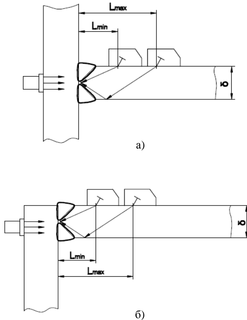
Рисунок 5.6 – Схемы прозвучивания корня шва на отсутствие непровара:
