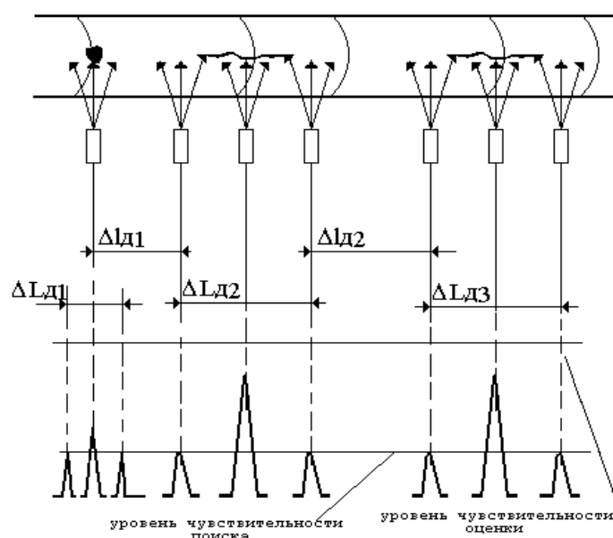
Рисунок 8.1 – Схема измерения \Delta L_d и \Delta l_d
