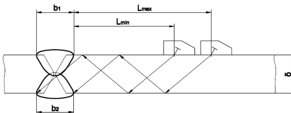
Рисунок 5.3 – Схема прозвучивания стыкового СС двукратно отраженным лучом ( m=2 ) с одной стороны одной плоскости
