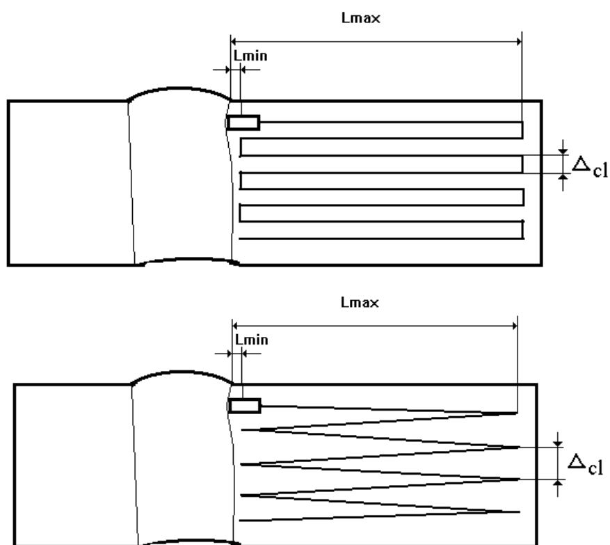
Рисунок 5.11 – Варианты схем поперечно-продольного сканирования
