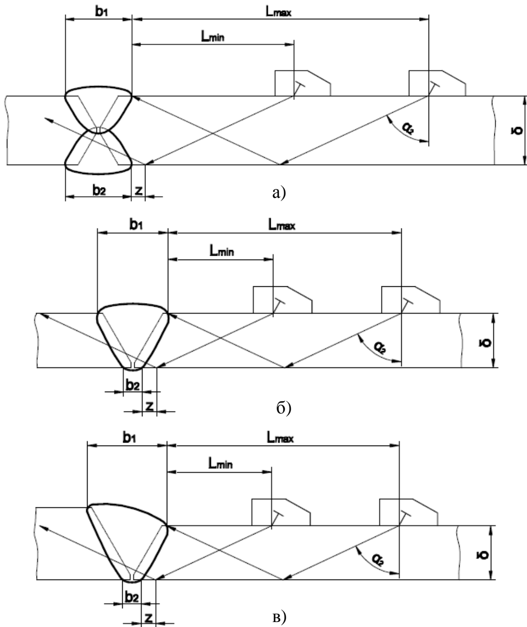
Рисунок 5.2 – Схема прозвучивания стыкового СС однократно отраженным лучом ( m=1 ) с одной стороны одной плоскости для швов с:
