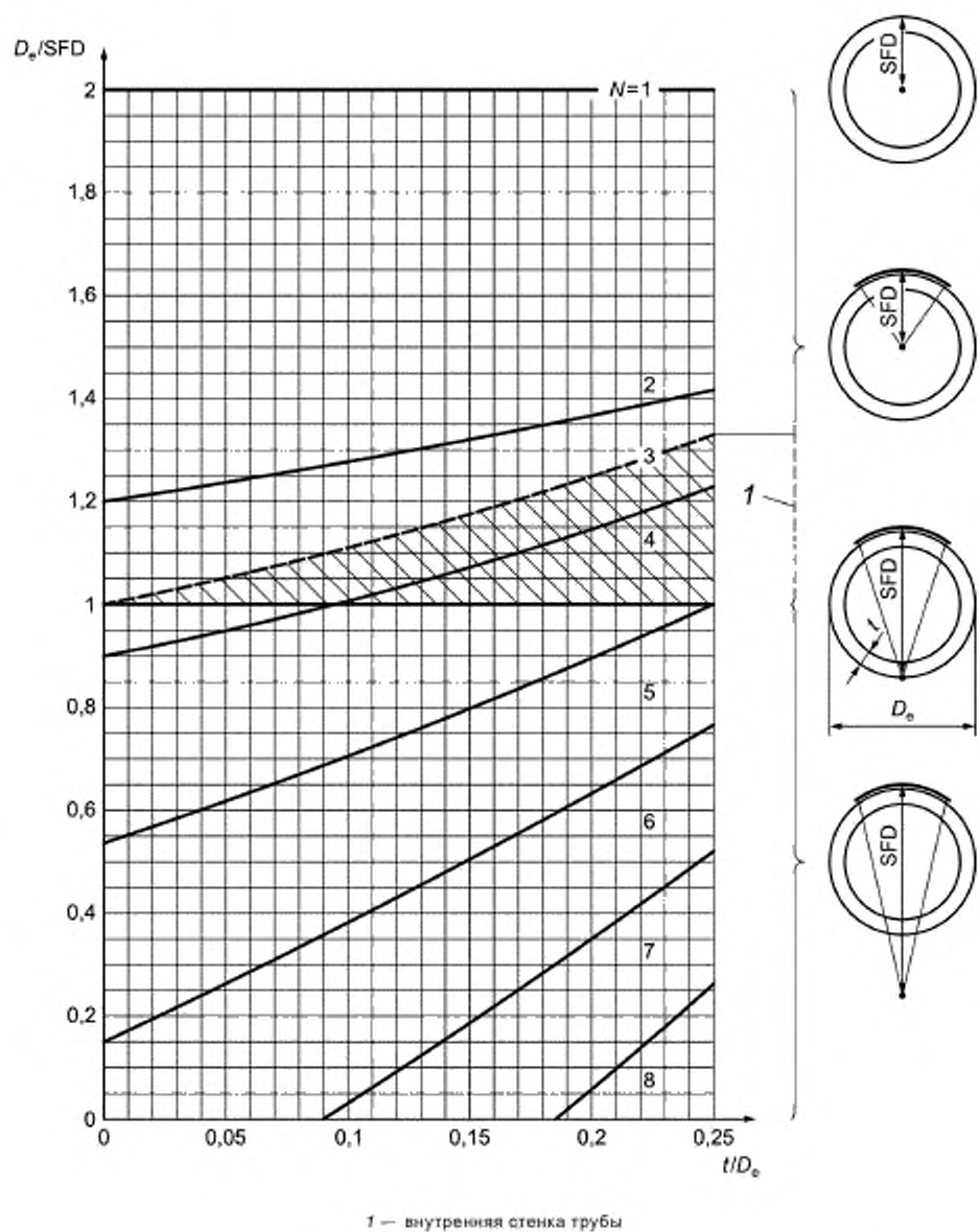
Рисунок А.4 — Минимальное количество экспозиций N при эксцентричном просвечивании с источником излучения внутри, а также при просвечивании через две стенки, при максимально допустимом увеличении просвечиваемой толщины \Delta t из-за наклонного направления излучения в проверяемой области равном 20 % (класс А), как функция отношений t/D_e и D_e/SFD
