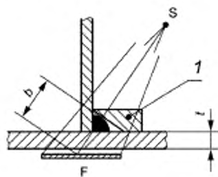
б) Схема контроля с краевым компенсатором
