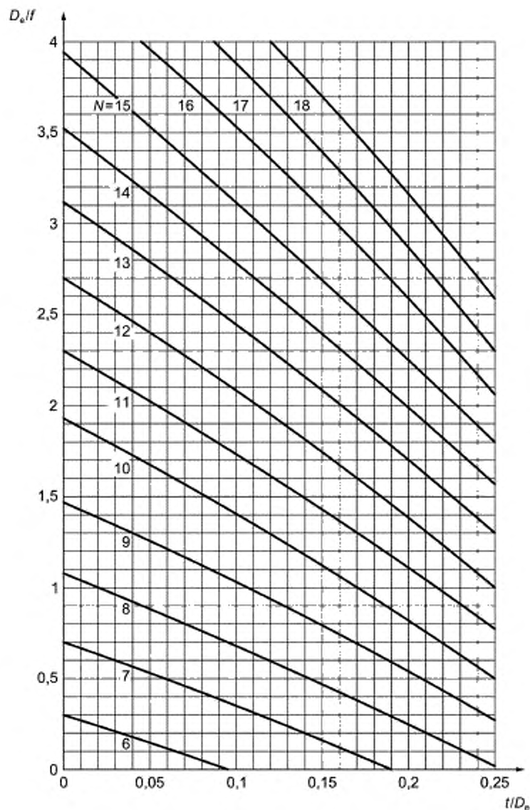
Рисунок А.3 — Минимальное количество экспозиций N при просвечивании через одну стенку с источником излучения снаружи при максимально допустимом увеличении просвечиваемой толщины \Delta t/t из-за наклонного направления излучения в проверяемой области равно 20 % (класс А), как функция отношений t/D_0 и D_0/f
