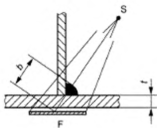
а) Схема контроля без краевого компенсатора
