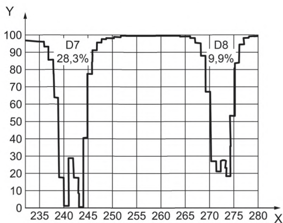
c — Увеличенный профиль проводочных пар D7 и D8
