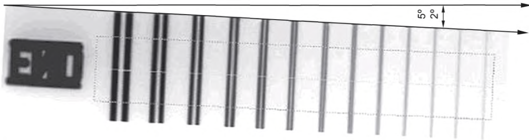
a — Изображение на радиографическом снимке (радиограмме) IQI двухпроводочного типа
